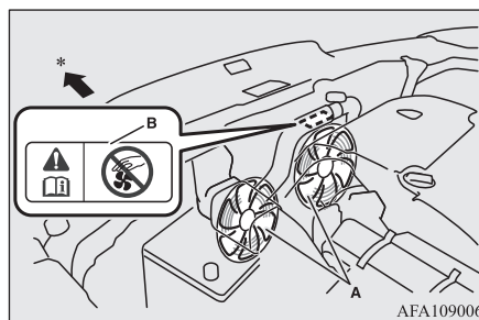
A- Koelventilatoren B- Waarschuwinglabel
